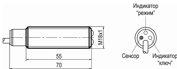
Рисунок 1 - Габаритный чертёж
